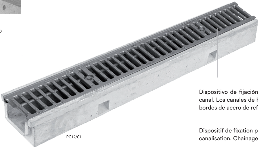
Bordes reforzados en acero Chaînage des blocs béton reinforced steel edges
