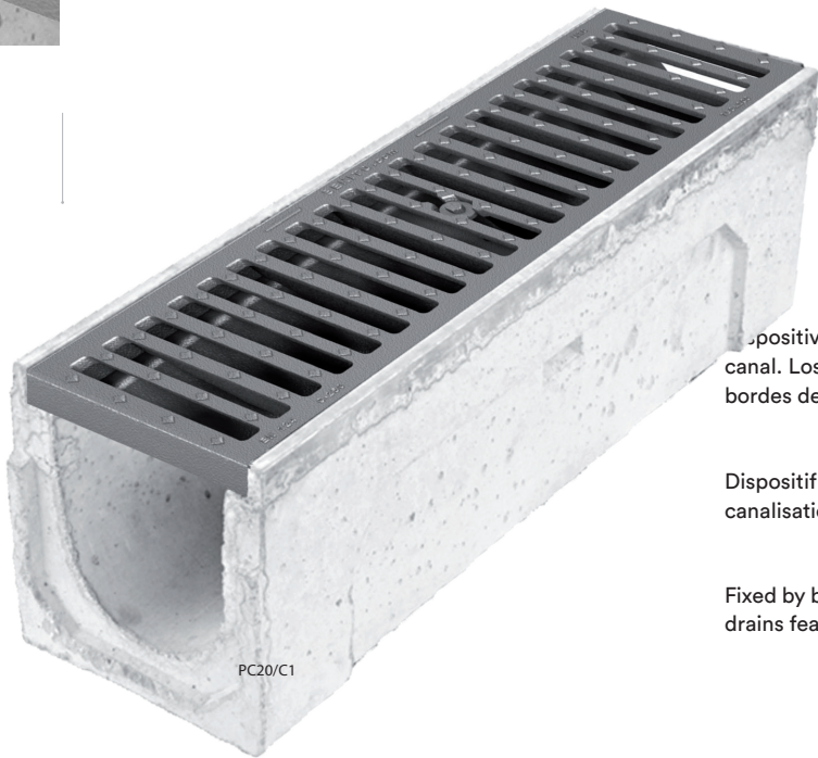
Bordes reforzados en acero Chaînage des blocs béton reinforced steel edges
